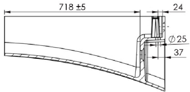
B-B
